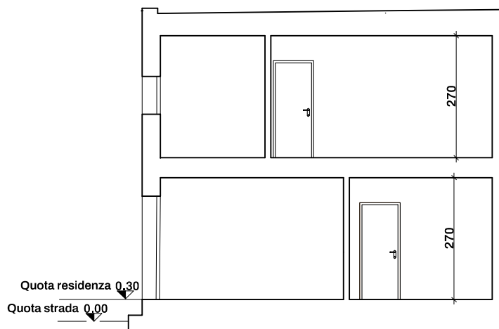
SEZIONE B-B'
