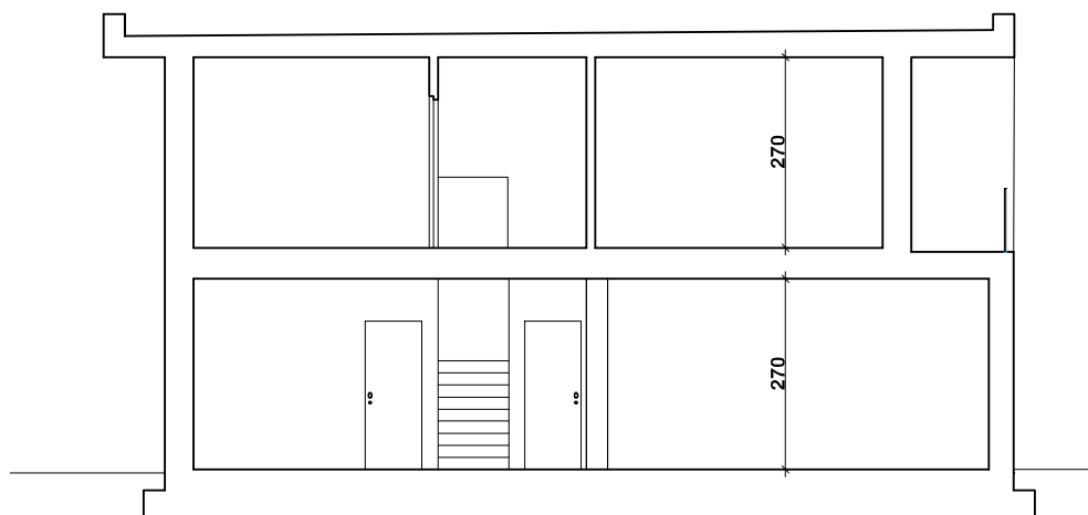
SEZIONE A-A'
