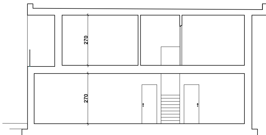
SEZIONE A-A'
