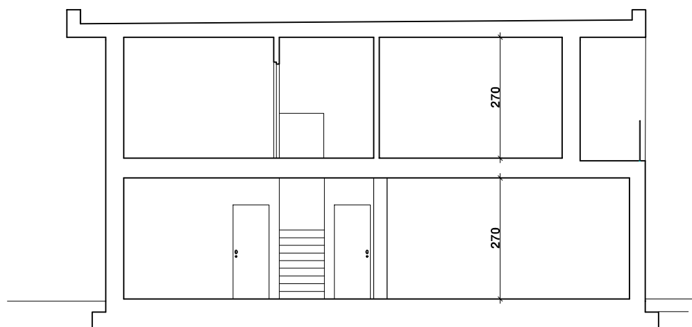
SEZIONE A-A'
