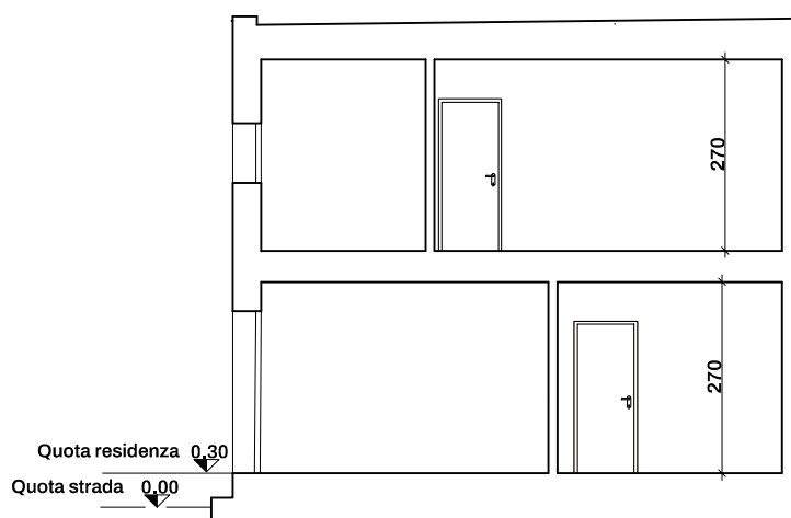
SEZIONE B-B'
