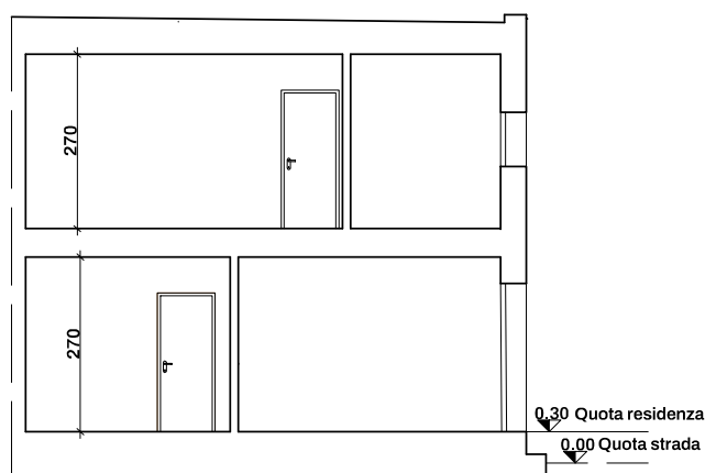
SEZIONE B-B'
