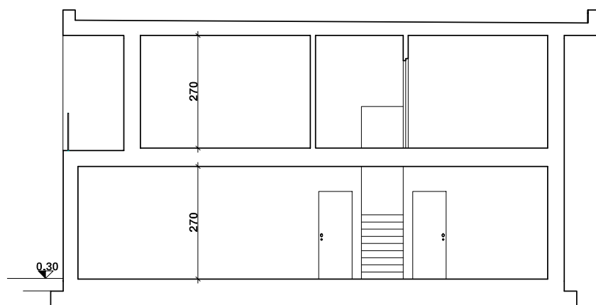
SEZIONE A-A'
