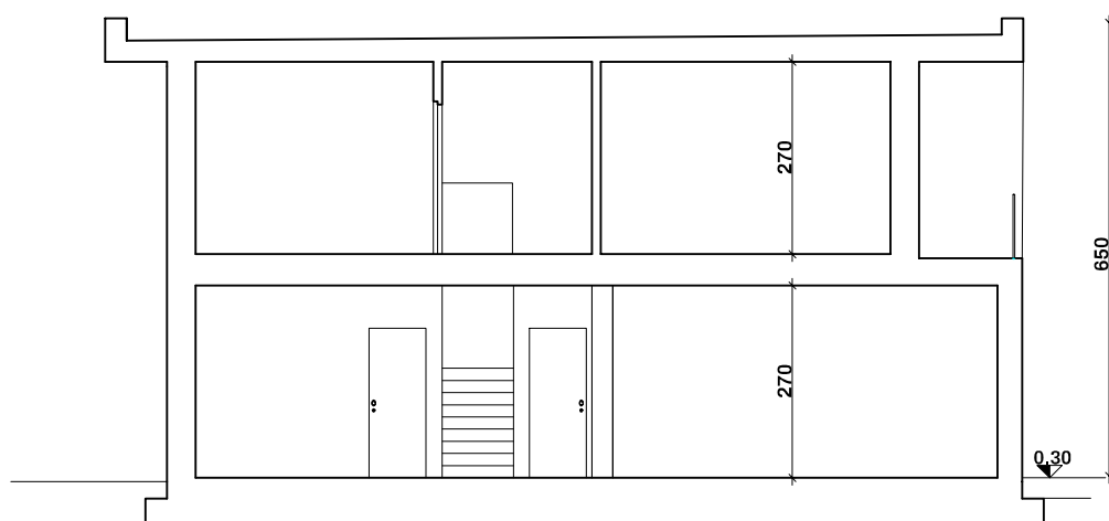
SEZIONE A-A'
