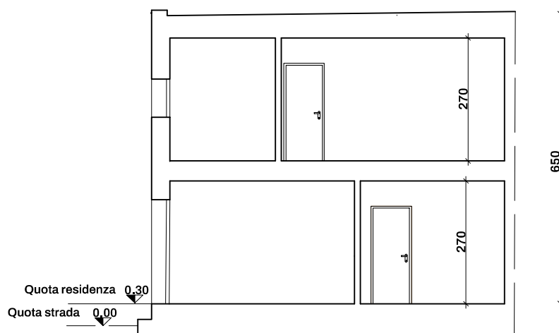
SEZIONE B-B'
