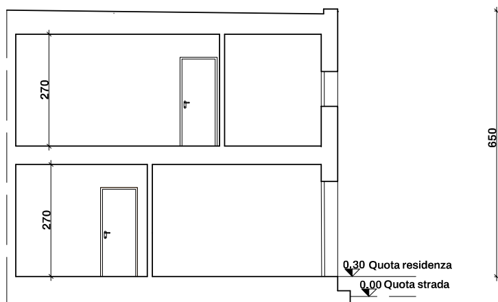
SEZIONE B-B'
