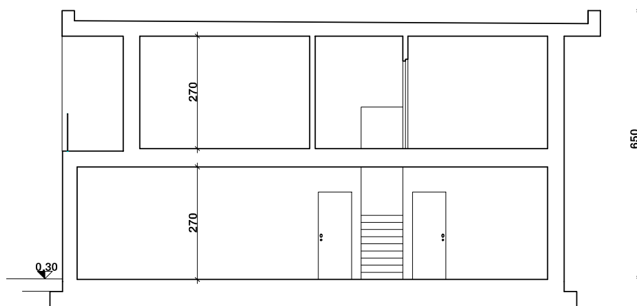
SEZIONE A-A'
